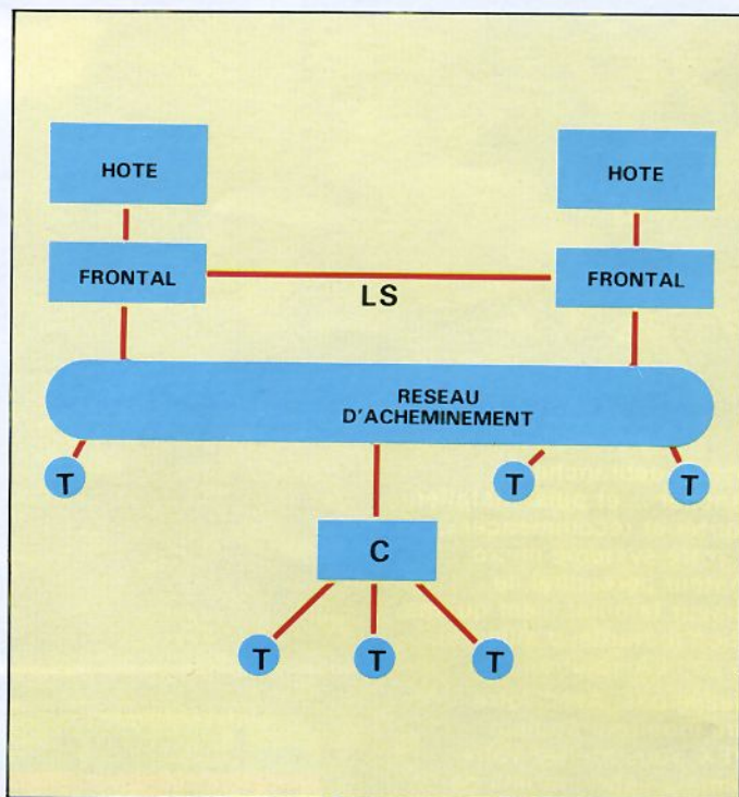
Fig. 1. - Schéma technique type d'un réseau SNA « classique ». Les ordinateurs « hôtes » contrôlent tout le réseau, via des machines « frontales » auxquelles sont sous-traitées les procédures de liaison. Une ou des liaisons spécialisées (LS) peuvent exister entre ces ordinateurs. Les terminaux (T) entrent exclusivement en relation avec ces ordinateurs, directement ou indirectement via des concentrateurs (C). Toute relation entre terminaux passe par au moins un ordinateur-hôte.
