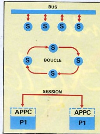
Fig. 3. - Session SNA « new-look ». Mieux adaptée aux échanges entre stations toutes « intelligentes », notamment quand elles sont interconnectées sur un pied d'égalité par un réseau local en bus ou en boucle. Des programmes (P1, P2) établissent entre eux des chemins de données selon des modalités normalisées par les logiciels APPC. Et sans en référer à une quelconque « autorité ».
