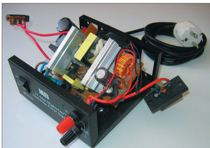
1 – L'alimentation avant modifications.
