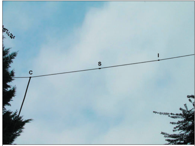
5 - Doublet raccourci (vue partielle).
