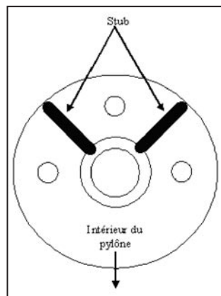
Schéma n° 6: Soudage de stub en renfort.
