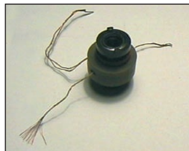
Figure 3: Bobinage HF formé de fil multibrin.
