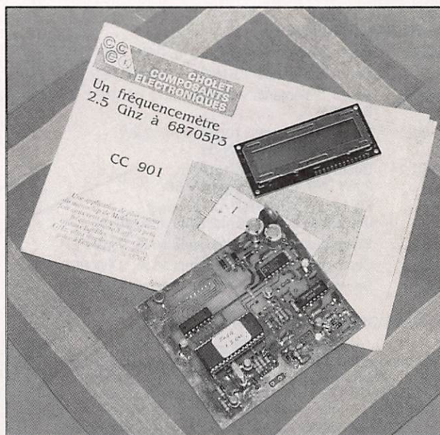
Fréquencesmètre 2,5 GHz.
