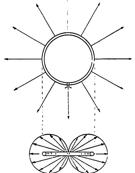
Rayonnement maxi dans le plan du cadre. 90^\circ = angle d'ouverture à 3 dB. Figure 6
