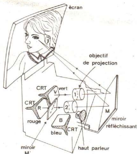
Fig. 5. Projecteur Sony.
