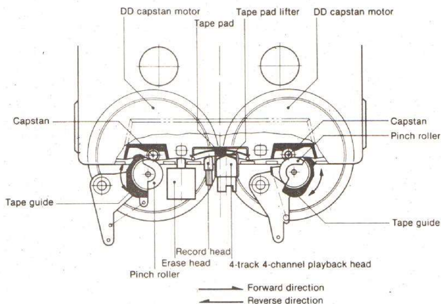
Fig. 4. — Dispositif autoreverse à double cabestan et entraînement direct (doc. Nakamichi).
