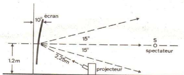
Fig. 4. - Installation du projecteur Super Color 9000.
