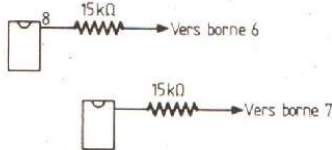
Fig. 5. - Branchement sur XR L 567.
