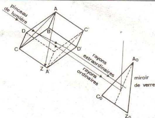
Fig. 8. — Le faisceau tombe normalement sur la face principale d'un cristal de spath.
