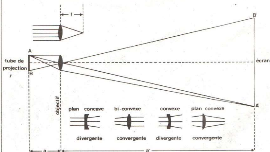
Fig. 3. — Emploi d'un objectif à quatre lentilles.
