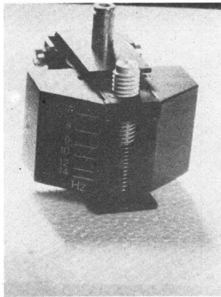
Fig. 8. — Encore le contrepoids et son étrier, mais vus du côté portant l'échelle des coefficients d'amortissement (0 à 3) notés « Q ». La valeur de Q utilisée se lit face à la pointe de l'aiguille centrale fileté, réglable au travers de l'axe de la molette, avec un petit tournevis d'horloger (un exemple figure parmi les accessoires de la table de lecture).
