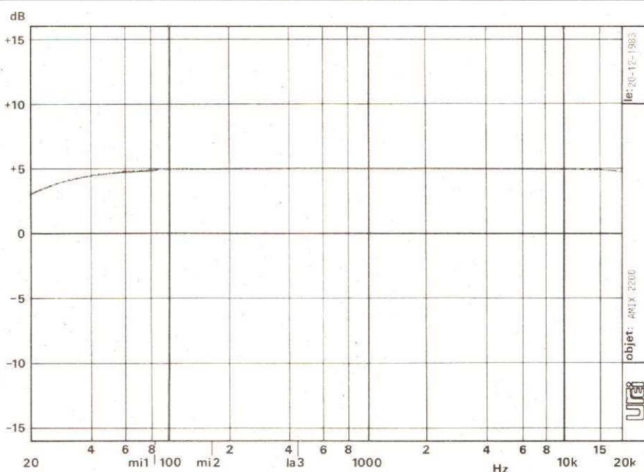
Courbe de réponse en fréquence de l'amplificateur AMIX 2200.
