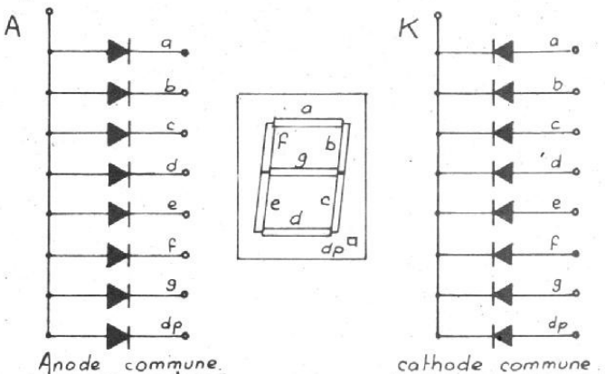
Fig. 9. — Afficheurs 7 segments.
