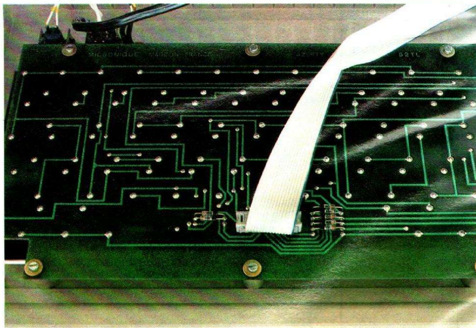
Le circuit imprimé du clavier et son câble plat de raccordement.
