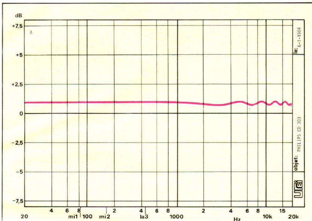
Courbe A. - L'allure de cette courbe de réponse en fréquence dont l'échelle verticale est particulièrement dilatée montre l'excellente linéarité moyenne de la courbe. On notera bien sûr l'ondulation traditionnelle propre aux filtres utilisés. Ici, nous avons une courbe qui tient dans une fourchette de 0,4 dB, soit \pm 0,2 dB, alors que le constructeur en annonce 0,3. Nous avons tracé ici la courbe de chacune des voies et constaté leur superposition parfaite.
