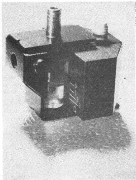
Fig. 7. — Contrepoids et son étrier isolés, vus du côté ressort et vis de réglage. La graduation de la partie mobile du contrepoids situe entre 7 et 14 Hz la fréquence de résonance propre de l'amortisseur, face à l'extrémité inférieure de la vis de réglage.
