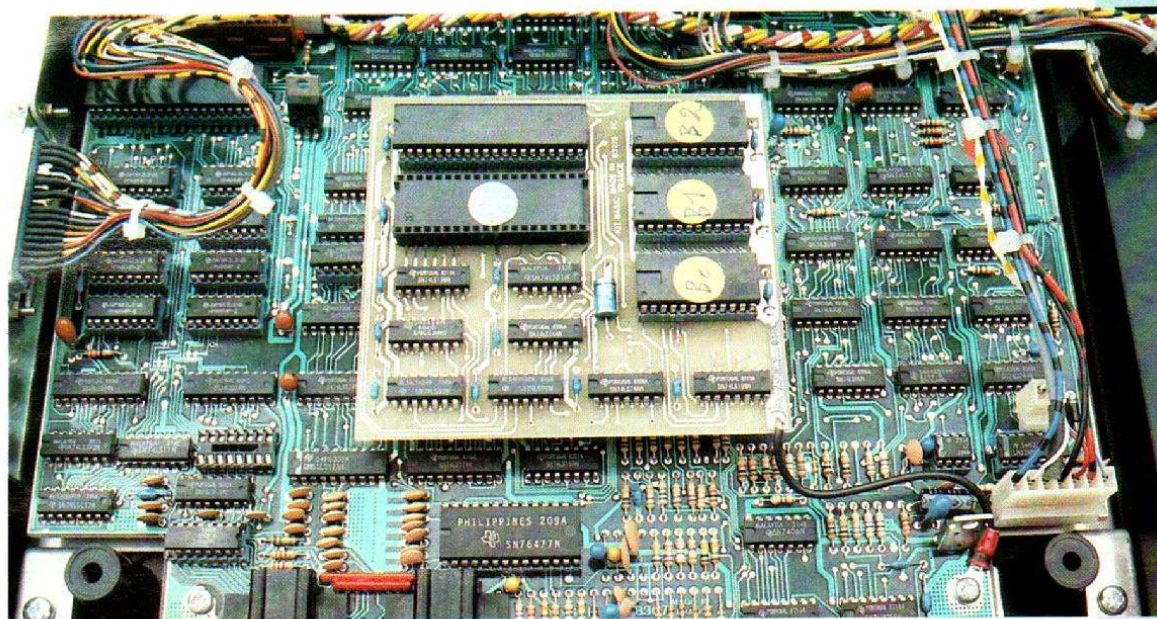
Le circuit imprimé principal.
