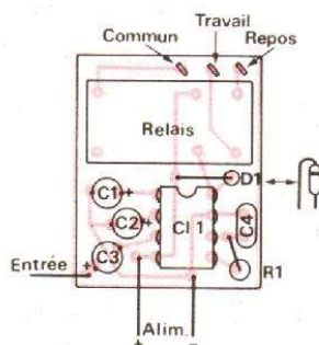
Fig. 3. - Implantation des composants.
