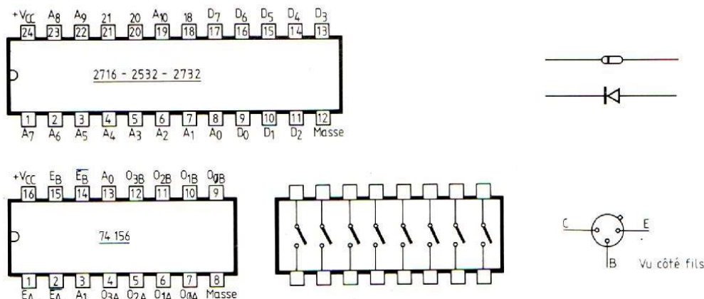
Fig. 6. — Brochage des éléments utilisés.
