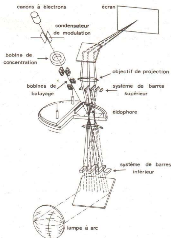
Fig. 6. - Aspect et schéma optique d'une projection suivant le procédé Eidophore.
