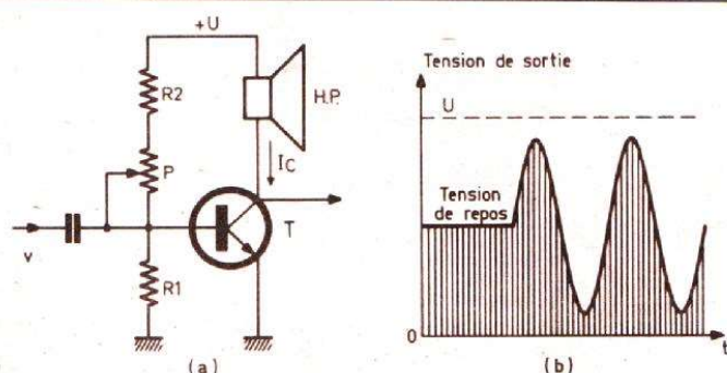
Fig. 1. — Schéma d'un amplificateur classe A (a) et représentation de la tension de sortie (b).
