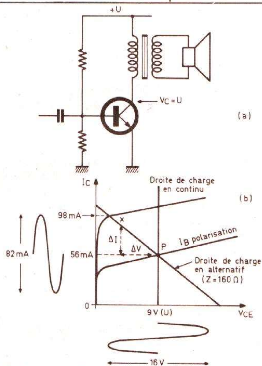
Fig. 5. — Amplificateur classe A chargé à travers un transformateur (a) et sa droite de charge (b).
