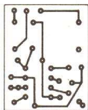
Fig. 2. - Le circuit imprimé (échelle 1).
