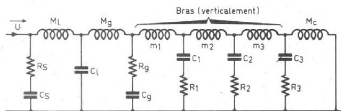
Fig. 3. — Modélisation élémentaire (ancienne analogie Olson) verticale, du bras NAD. U est la vitesse imposée par la gravure du sillon, d'élasticité C_s ( 2.10^{-2} \mu\text{m/mN} , environ) ; R_s la résistance de la matière du sillon ; M_1 , la masse du levier porte-pointe ; C_g , son élasticité propre ; M_g , la masse de l'équipage mobile, d'élasticité C_g et de résistance R_g ; le bras souple est schématisé sous forme d'une ligne, formée de cellules élémentaires ( m_1, c_1, r_1, \dots ) ; enfin M_c est la masse de contrepoids sans son amortisseur (le tout, vu de la pointe de lecture).
