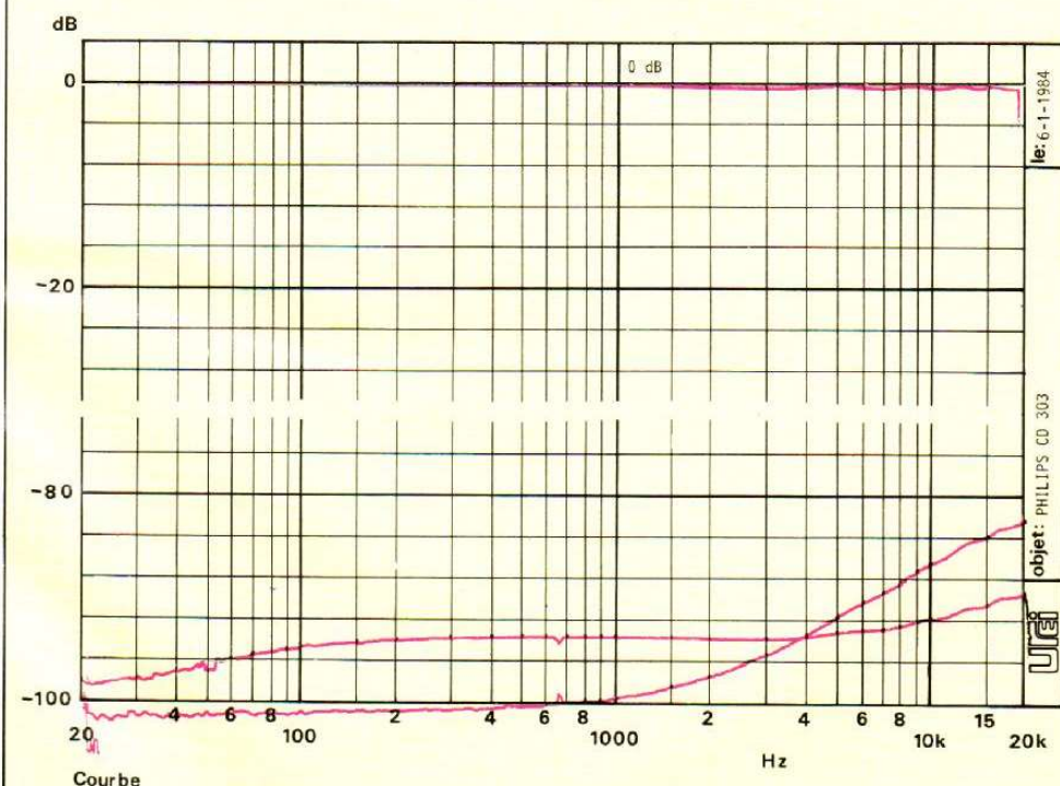
Courbe B. - Tout en haut, nous avons la courbe de réponse en fréquence pratiquement confondue avec une ligne horizontale placée à 0 dB. La diaphonie a un niveau excellent avec, en particulier pour l'une des deux voies, un niveau meilleur que 100 dB, ce que nous n'avons jamais rencontré. Cette diaphonie est en fait celle des circuits audio analogiques, câble compris.
