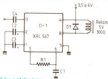
Fig. 1. — Schéma théorique.
